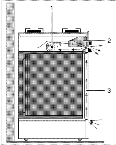
1 Soğutma fanı
